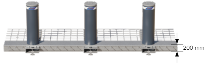
Standard-Bodenbefestigung mit drei feststehenden Zylindern
