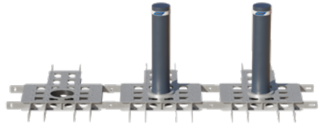
Konfiguration mit zwei feststehenden Zylindern
